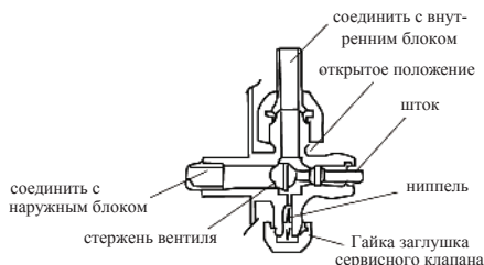
трехходовой вентиль
